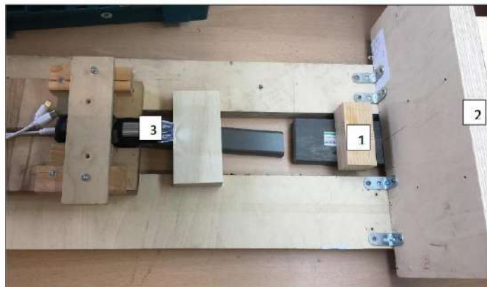
Figure 4 : Support pour les mesures d'imprégnation et de tension de surface.
